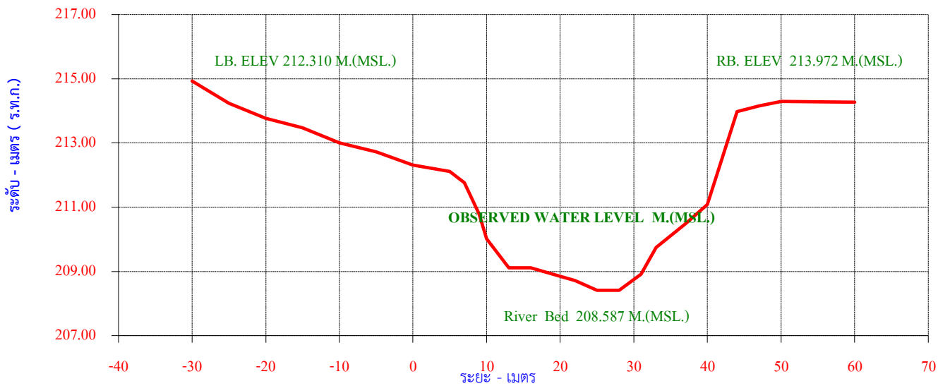
รูปตัดขวางลำน้ำ ปีน้ำ 2566 สถานี N.39 น้ำปาด อ.ปากท่า จ.อุตรดิตถ์
